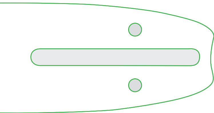
ANSCHLUSS: A041, Z041 Dolmar, Makita, Echo und andere 3/8" LP 1,1 mm und 1,3 mm
